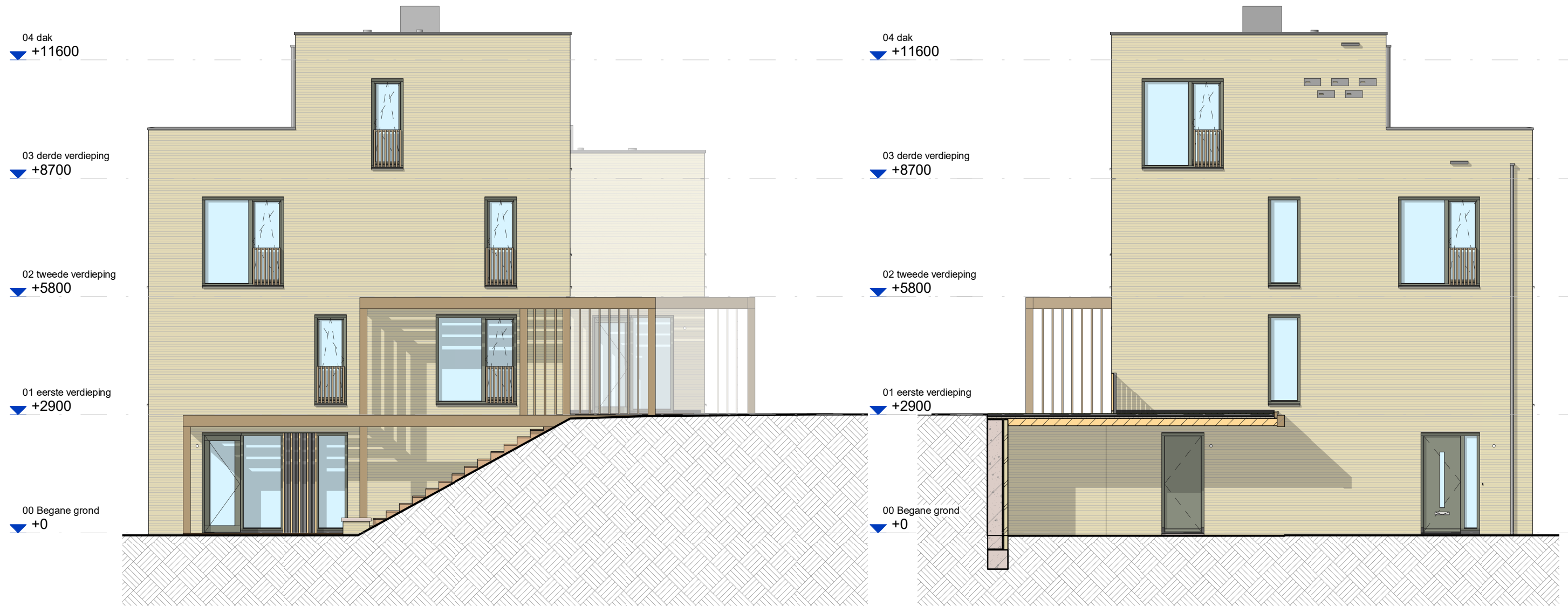
Rechter zijgevel
