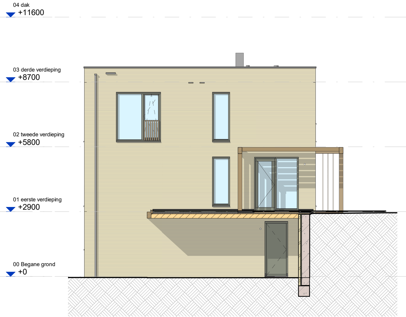
Rechter zijgevel
