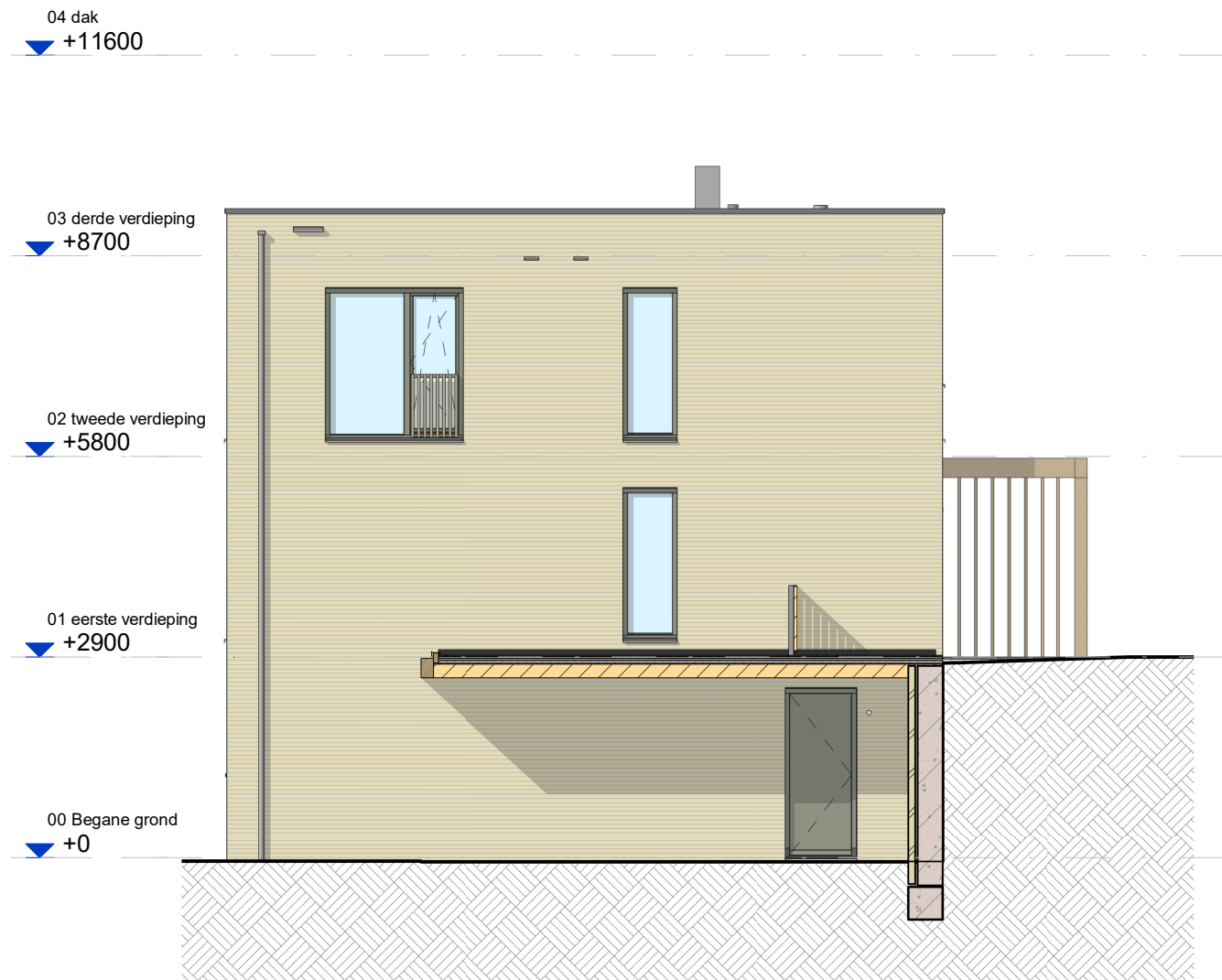
Rechter zijgevel
