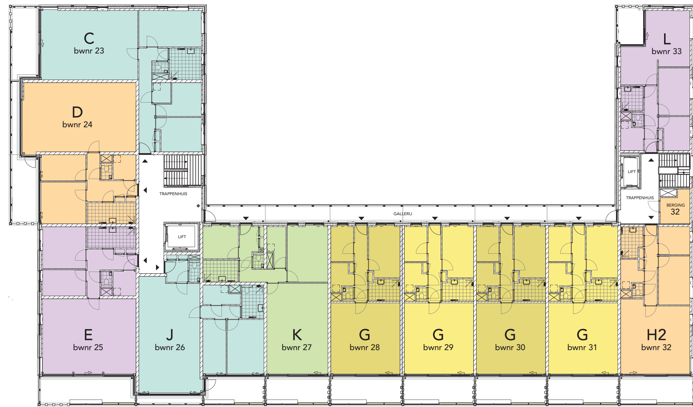
TWEEDE VERDIEPING
