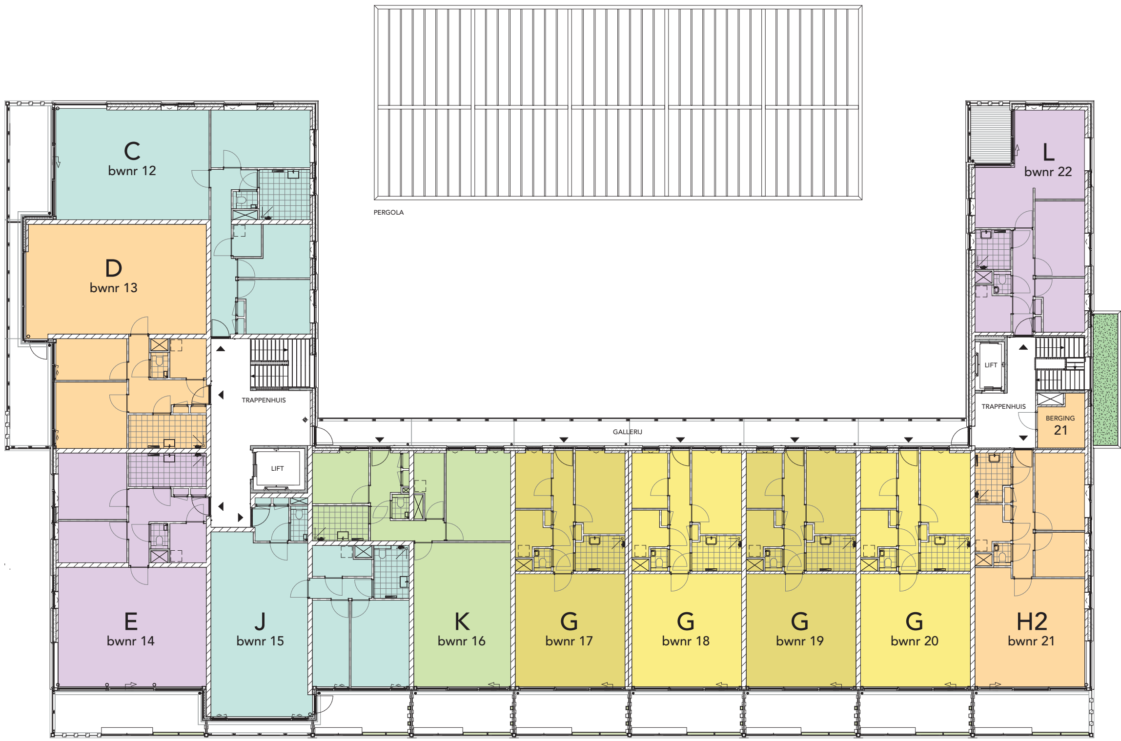
EERSTE VERDIEPING
