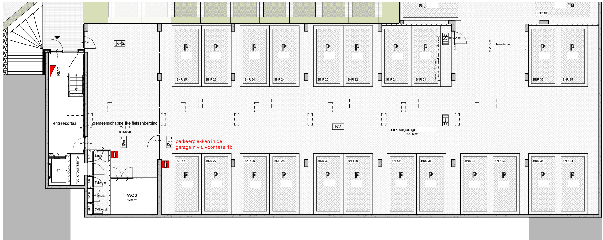
Plattegrond parkeerkelder 1 : 100
