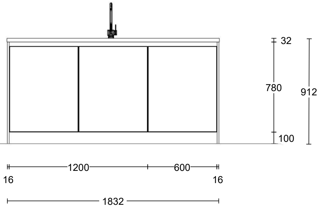
Vooraanzicht eiland
