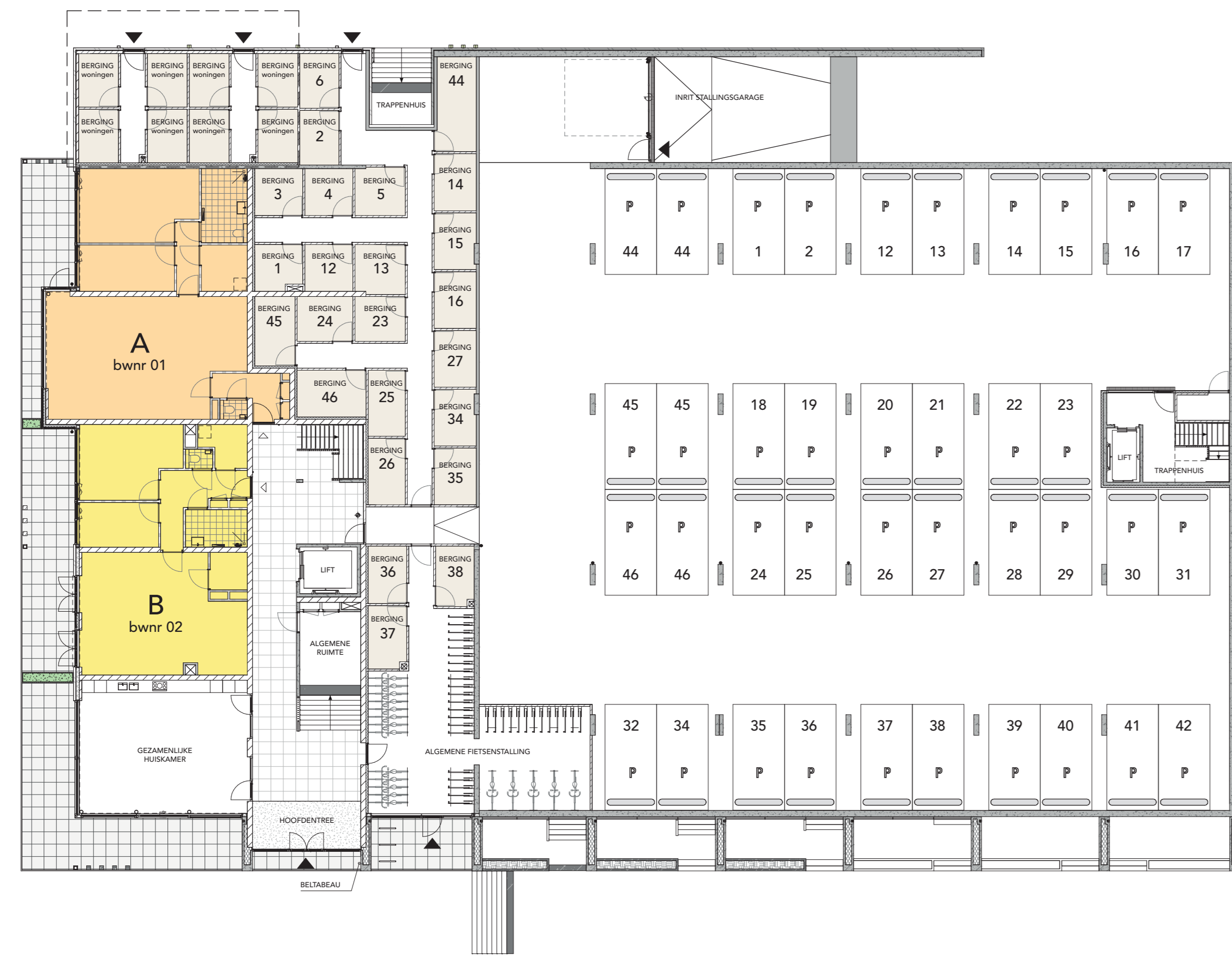
LAAG -1
