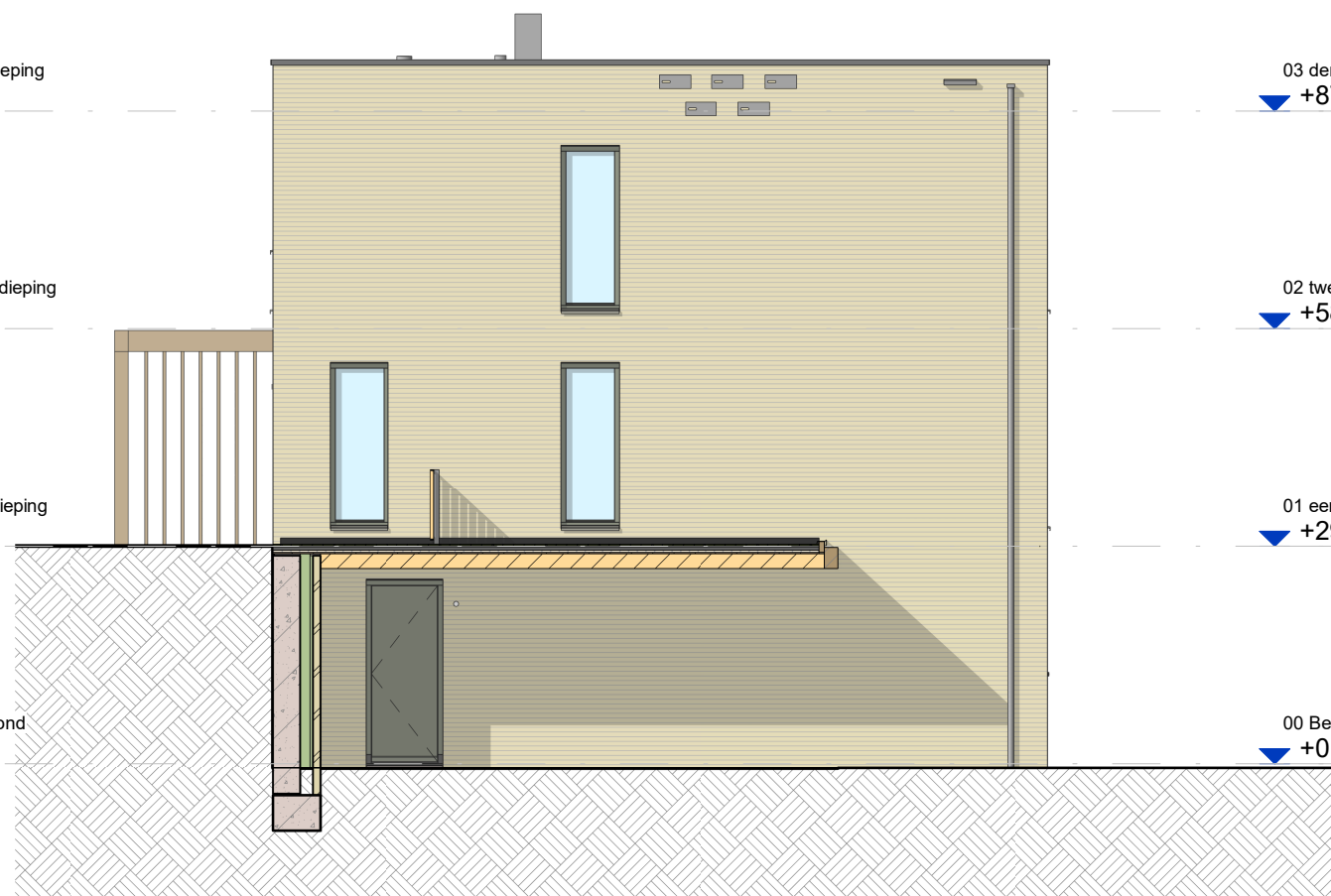
Linker zijgevel
