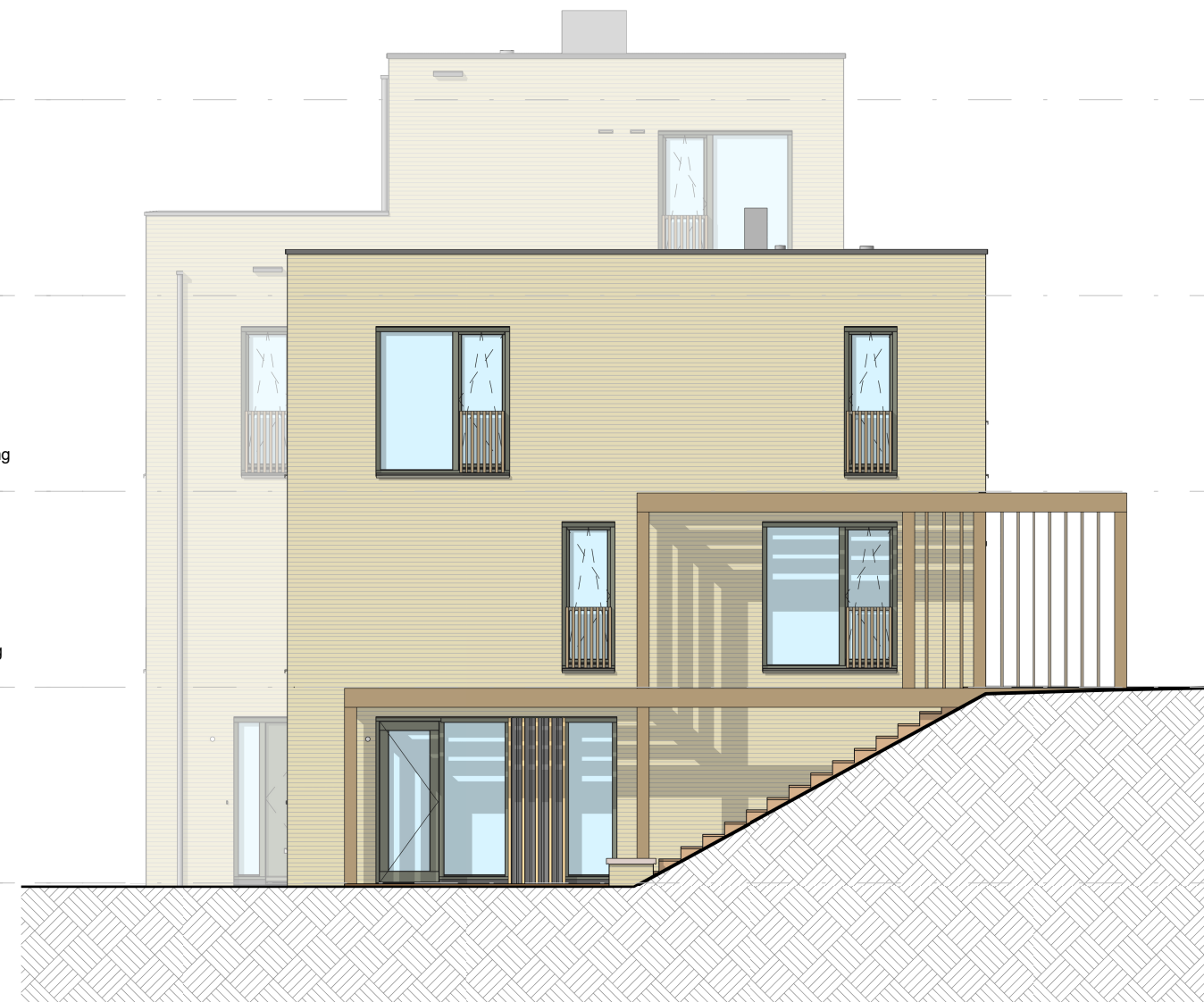
Rechter zijgevel
